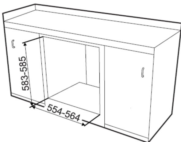
Вграждане под работните плотове(мм)
