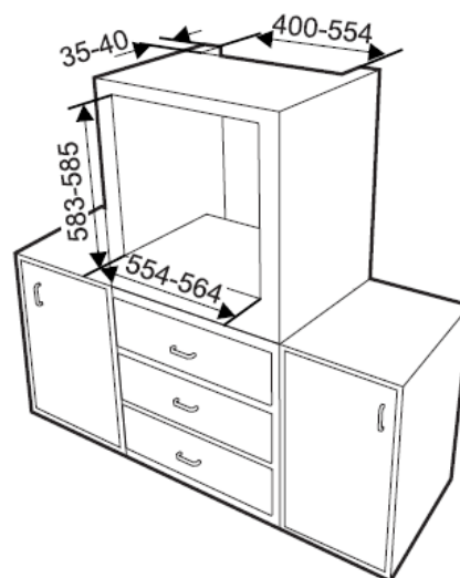
Вграждане в колона(мм)
